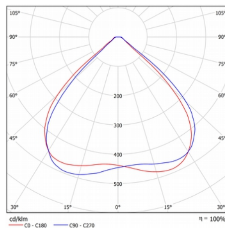
lens: socz-90x90
