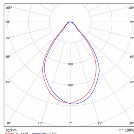
lens: socz-60x60
